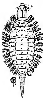
Fig. 239. Brachypsectra fulva Lec.
